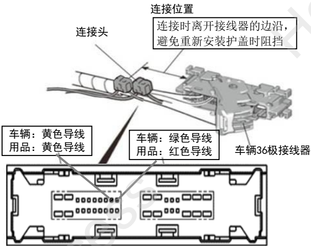
<从线束侧的视图>
